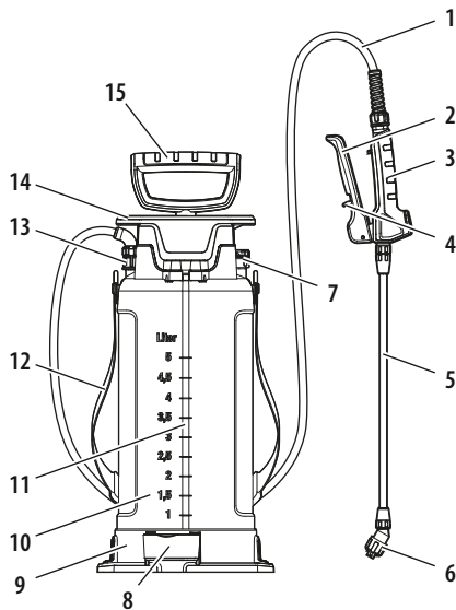
Teile des Drucksprüngergeräts
